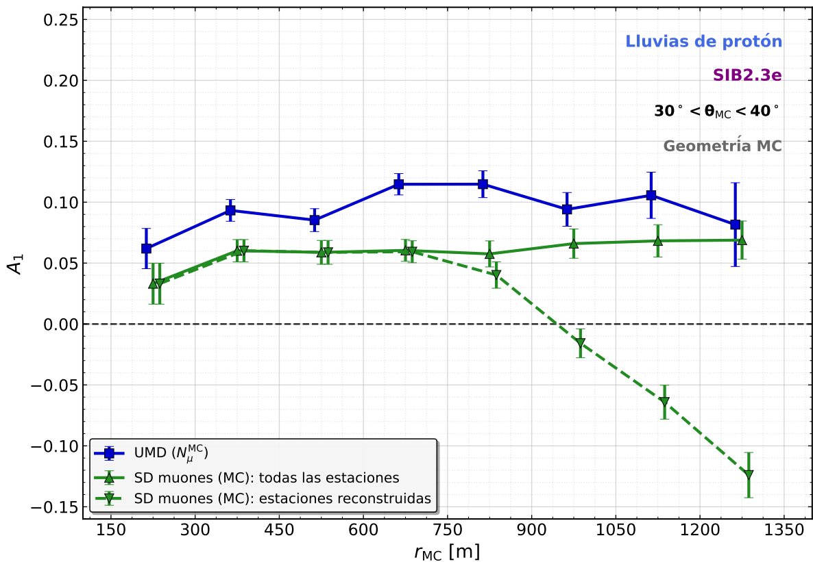
Figura 6.1.5: Asimetría del número de muones Monte Carlo del SD calculada sobre todas las estaciones simuladas y sólo sobre las que forman parte del evento reconstruido, junto con la del número de muones inyectado en el UMD ( N_{\mu}^{MC} ), para 30^\circ \leq \theta < 40^\circ y geometría Monte Carlo. Las barras de error se obtienen con un bootstrap sobre las lluvias de la muestra. La inversión del SD sólo aparece al restringir el promedio a las estaciones reconstruidas.
