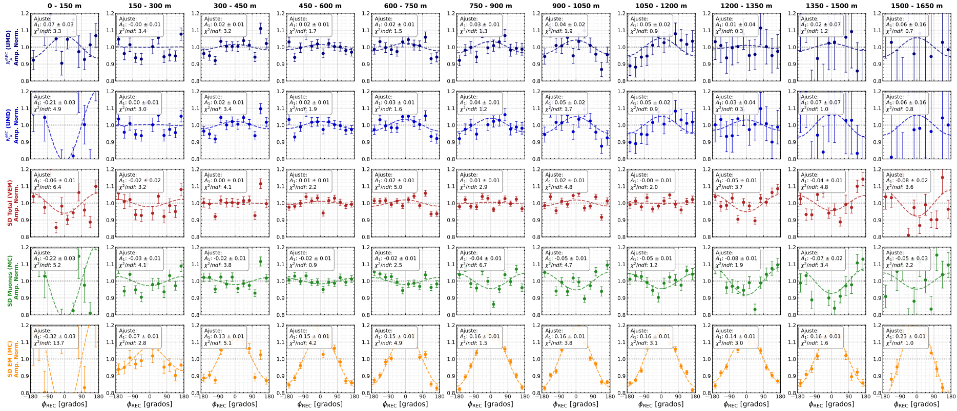
Figura C.2.2: Análisis multiseñal de asimetría azimutal usando la geometría Reconstruida para lluvias con ángulos cenitales verdaderos entre 10^\circ y 20^\circ . Las barras de error representan el error estándar de la media en cada bin angular.
