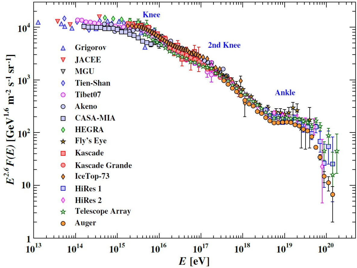
Figura 1.1.1: Espectro de energía de rayos cósmicos en los rangos de energía 10^{13} eV < E < 2 \times 10^{20} eV. Se observa cómo cambia el flujo escalado por E^{2.6} y se visualizan las características morfológicas más relevantes: la 'rodilla', la 'segunda rodilla', el 'tobillo' y la supresión de flujo a energías extremas. Obtenido de [9].
