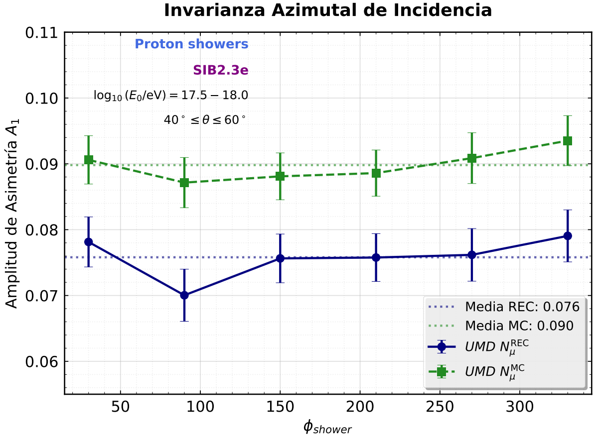
Figura 5.3.1: Amplitud A_1 en función del ángulo azimutal de la lluvia. Se observa la independencia del observable respecto a la dirección de arribo.
