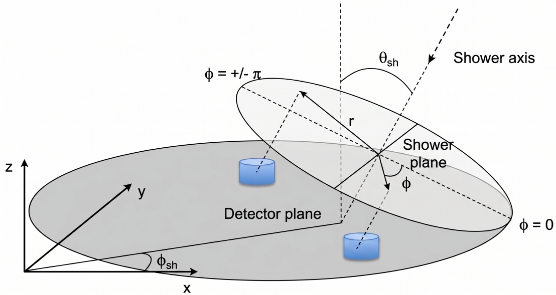
Figura 3.1.1: Esquema geométrico de una Lluvia Atmosférica Extensa (EAS) con ángulo cenital \theta_{sh} y azimut \phi_{sh} de arriba. Las posiciones de los detectores en el plano del suelo ( detector plane ) se proyectan sobre el plano de la lluvia ( shower plane ), perpendicular al eje, definiendo las coordenadas intrínsecas r y \phi . La región temprana corresponde a \phi = 0 y la tardía a \phi = \pm\pi . En el texto se denota \theta \equiv \theta_{sh} .
