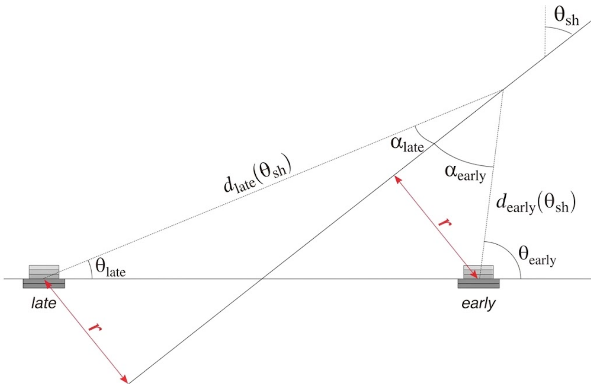
Figura 3.2.1: Esquema geométrico de la dispersión de las partículas en una lluvia de ángulo cenital \theta_{sh} , para un punto de producción sobre el eje. Debido a la inclinación, para alcanzar un mismo radio r en el plano de la lluvia, la región tardía ( late ) requiere un ángulo de emisión \alpha_{late} menor que la región temprana ( early ), \alpha_{early} , y se encuentra a mayor distancia del punto de producción ( d_{late} > d_{early} ). Los ángulos \theta_{early} y \theta_{late} se miden respecto del suelo; en el texto se utiliza el ángulo cenital local de cada trayectoria, medido desde la vertical, \vartheta = 90^\circ - \theta_{early} (o 90^\circ - \theta_{late} ), de modo que \vartheta_{temprano} < \vartheta_{tardio} . Adaptado de [19].
