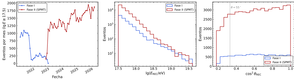
Figura 6.4.1: Muestra de datos de campo con \lg(E/\text{eV}) \geq 17,5 luego de los cortes de calidad. Izquierda: eventos por mes en cada flujo de reconstrucción. Centro: espectro de energía reconstruido. Derecha: distribución en \cos^2 \theta ; la línea vertical marca \theta = 55^\circ .
