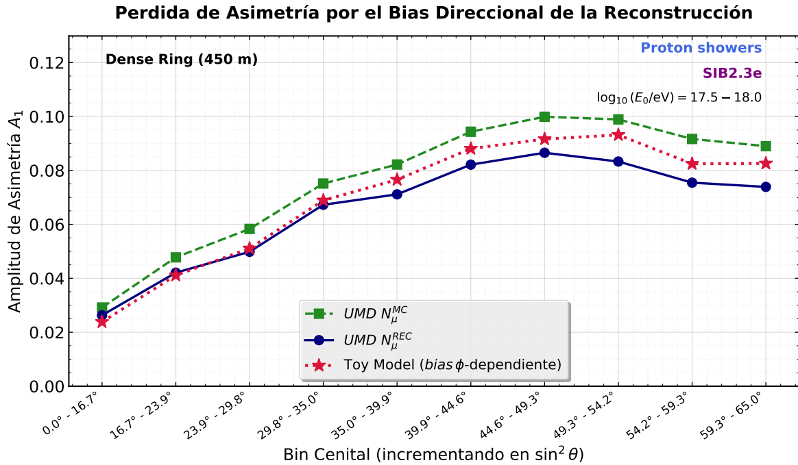
Figura 5.2.4: Comparación de la amplitud de asimetría A_1 para muones inyectados (verde), reconstruidos (azul) y el resultado del Toy Model direccional (rojo). Se aprecian dos regímenes diferenciados de degradación de señal según la inclinación de la cascada.
