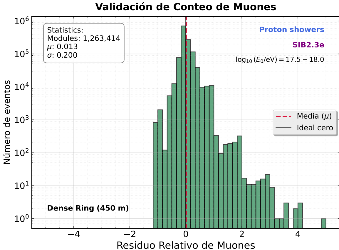
Figura 5.2.2: Distribución del residuo relativo en la reconstrucción de muones. Aunque la media es cercana a cero, se observa una asimetría intrínseca con una cola extendida hacia la sobre-reconstrucción de partículas.
