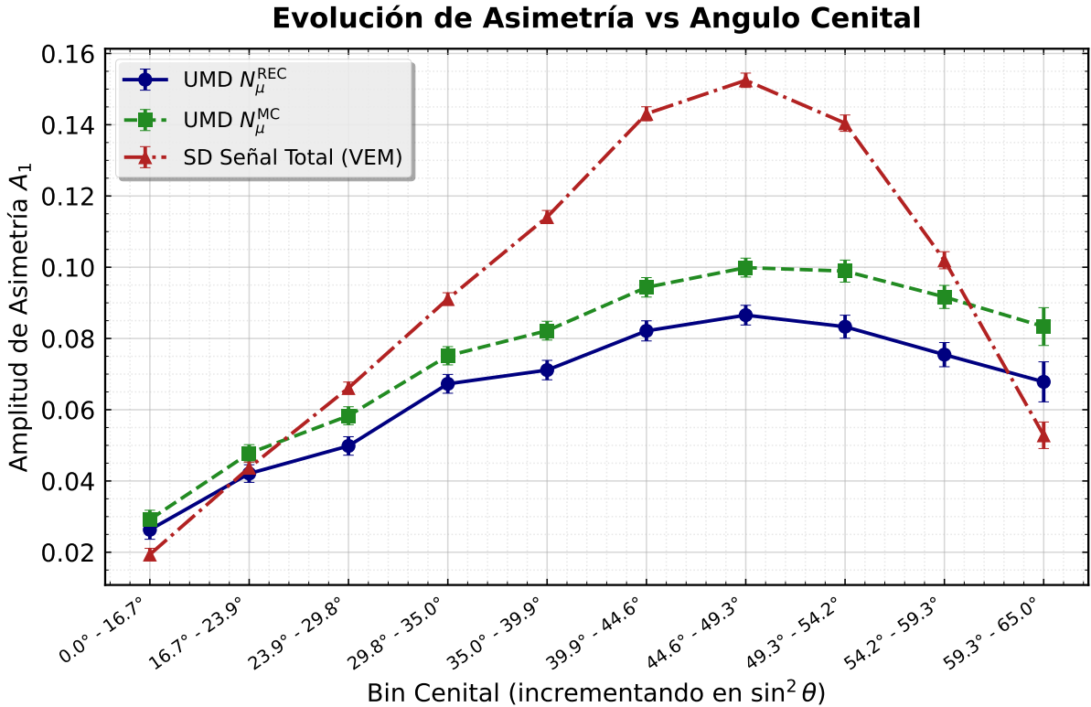
Figura 5.1.2: Evolución de la amplitud A_1 con su error en función de \theta para el UMD (REC en azul, MC en verde) y el SD (rojo). Se observa la inversión de dominancia entre el SD y el UMD a altas inclinaciones.
