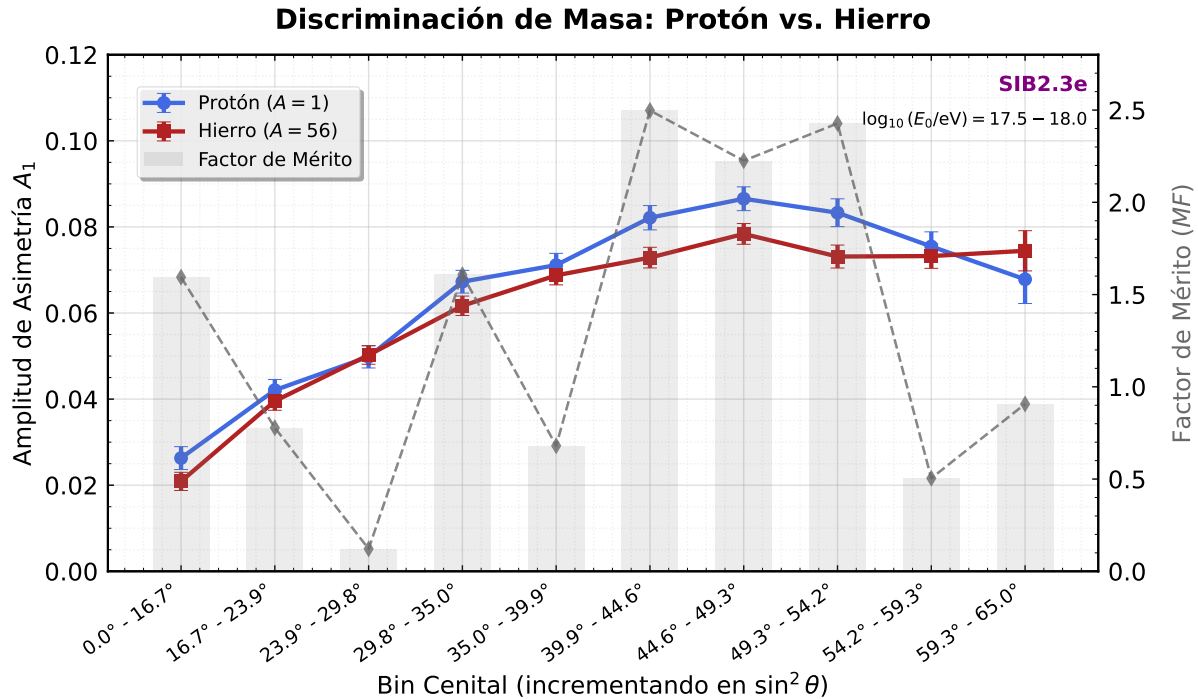
Figura 5.5.1: Evolución del Factor de Mérito ( MF ) en función del ángulo cenital. Se identifica un Sweet Spot de máxima separación entre bins de 40^\circ y 55^\circ , donde el poder de discriminación alcanza su máximo antes de degradarse por efectos instrumentales.
