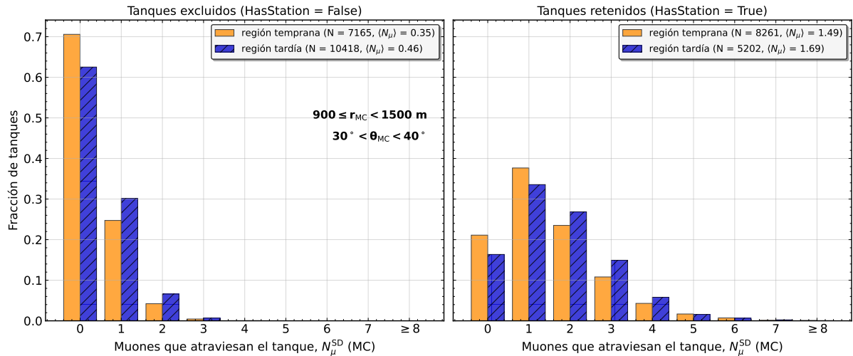
Figura 6.1.6: Distribución del número de muones Monte Carlo que atraviesan cada tanque del SD para las estaciones que quedan fuera del evento reconstruido (izquierda) y para las que forman parte de él (derecha), en las regiones temprana ( |\phi| < 60^\circ ) y tardía ( |\phi| > 120^\circ ). Lluvias de protón (SIBYLL 2.3e), 30^\circ \leq \theta < 40^\circ , 900 \leq r < 1500 m y geometría Monte Carlo. Cada distribución está normalizada a su número de tanques.
