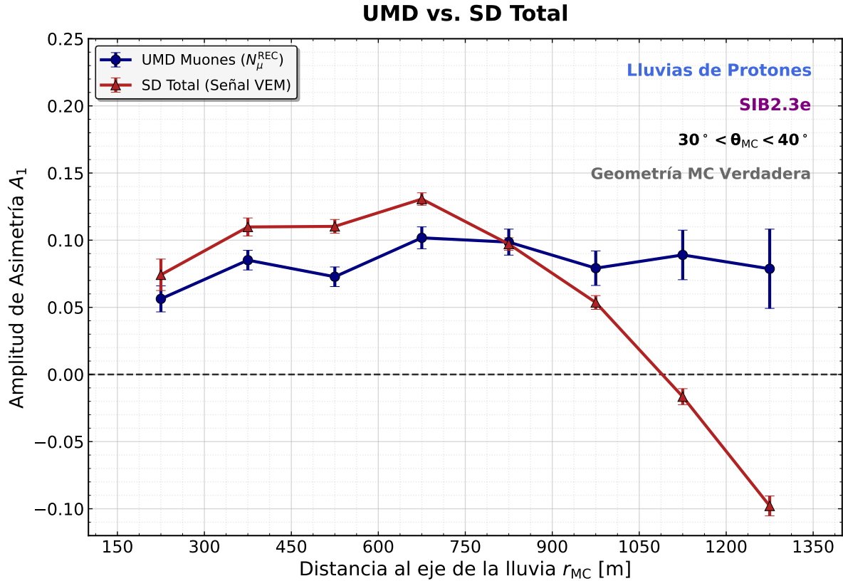
Figura 6.1.3: Comparación de la evolución radial de la amplitud de asimetría A_1 entre el número de muones reconstruido por el UMD ( N_{\mu}^{REC} ) y la señal total registrada por los tanques del SD en superficie, evaluada para el rango cenital de referencia de 30^{\circ} \leq \theta < 40^{\circ} . Ambas curvas fueron extraídas fijando la geometría real de Monte Carlo donde las barras de error representan el error estándar de la media. Se evidencia el comportamiento divergente de los observables: mientras que el UMD mantiene una asimetría positiva a todas las distancias, la señal del SD Total exhibe una severa disminución de la asimetría que culmina en una inversión (asimetría negativa) en el far-core .
