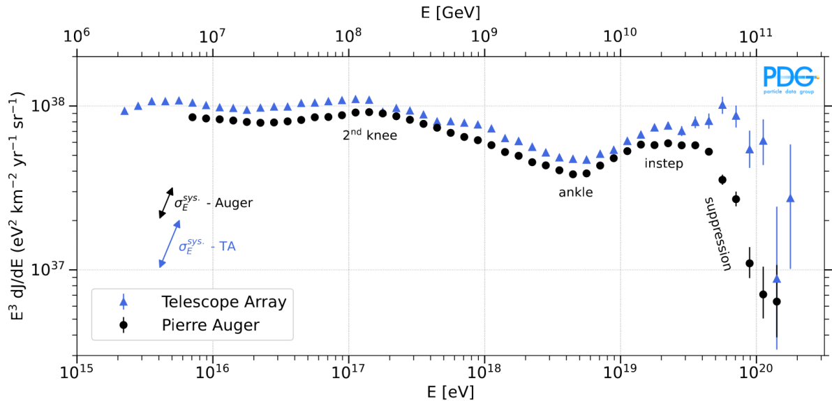
Figura 1.1.2: Espectro de energía de rayos cósmicos de ultra-alta energía obtenido a partir de los datos del Observatorio Pierre Auger y Telescope Array en el rango energético 2 \times 10^{15} eV < E < 2 \times 10^{20} eV. Se detalla la evolución del flujo escalado por E^3 y se evidencian las estructuras de alta energía: la 'segunda rodilla', el 'tobillo', el 'instep' y la supresión final del flujo. Obtenido de [8].
