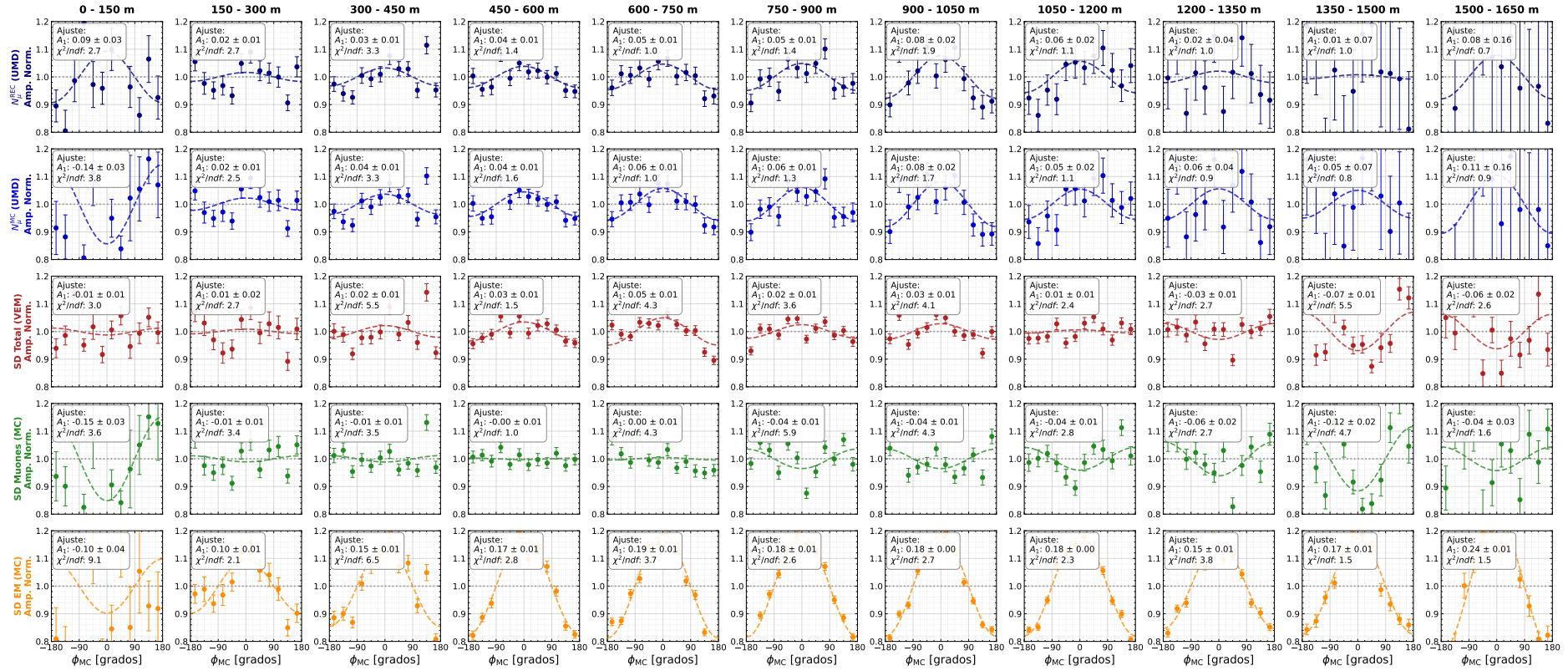
Figura C.1.2: Análisis multiseñal de asimetría azimutal forzando la geometría Monte Carlo para lluvias con ángulos cenitales verdaderos entre 10^\circ y 20^\circ .
