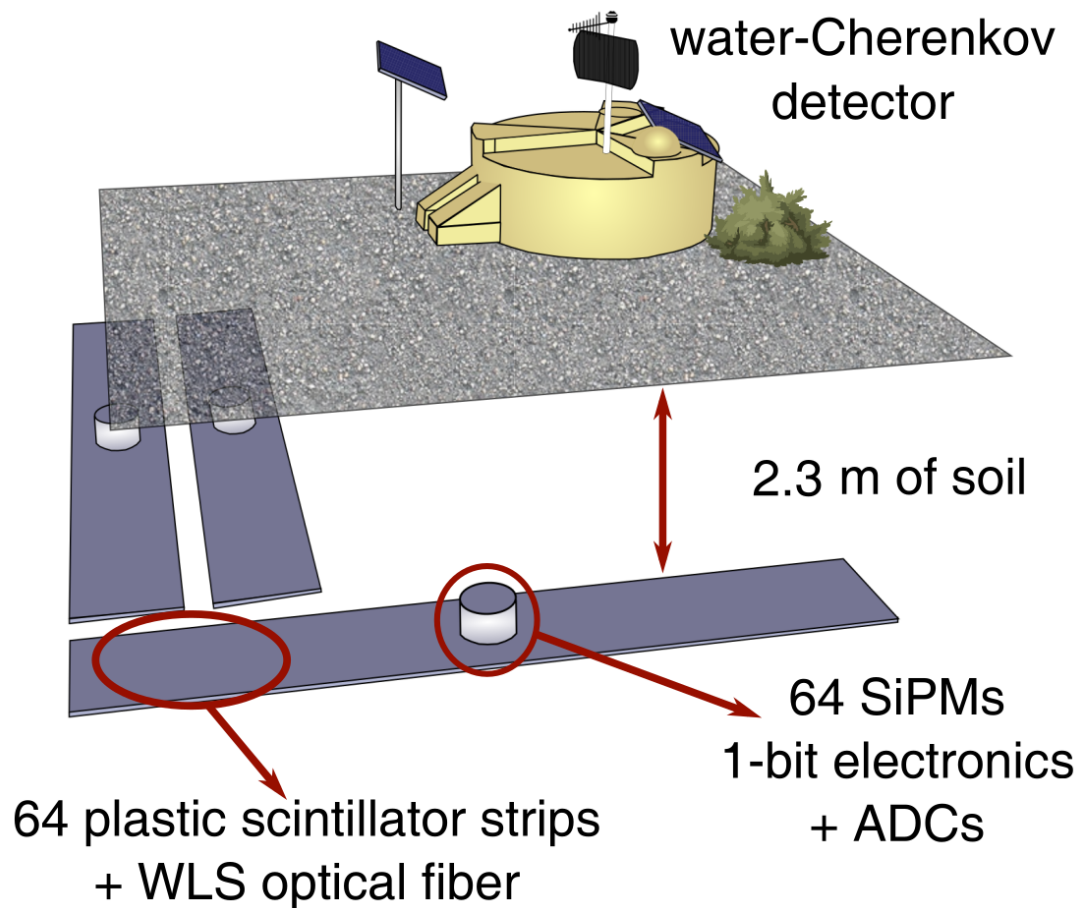
Figura 2.4.1: Esquema de Detector Subterráneo de Muones junto a su estación de superficie asociada donde se observa la distribución de los tres módulos centelladores. Obtenido de [13].
