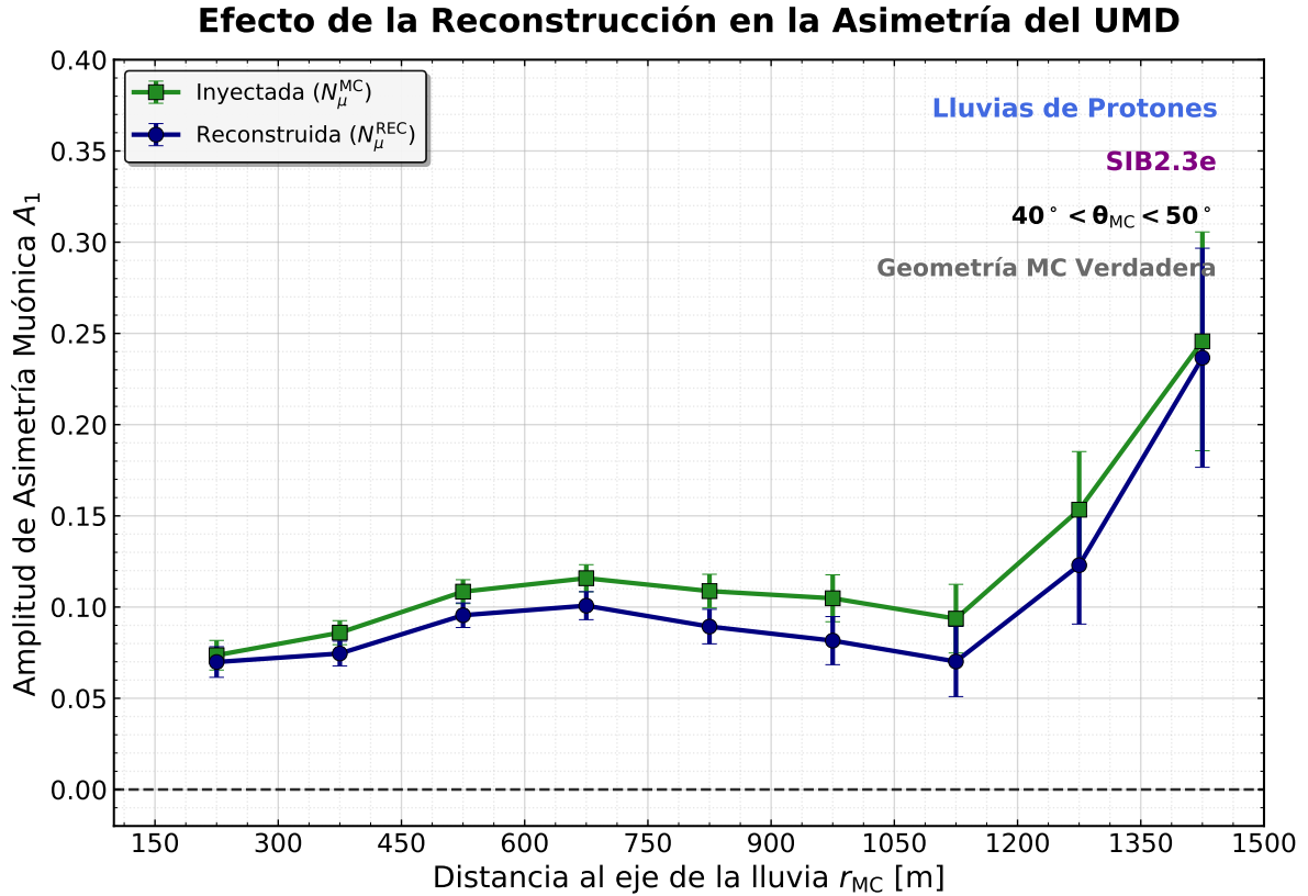
Figura 6.1.2: Comparación de la amplitud de asimetría A_1 obtenida a partir del número de muones inyectado ( N_{\mu}^{MC} ) frente al número de muones reconstruido ( N_{\mu}^{REC} ) para el rango cenital de referencia de 40^{\circ} \leq \theta < 50^{\circ} . Ambas se realizan fijando las coordenadas a nivel Monte Carlo. Se observa que la respuesta instrumental del detector introduce una atenuación sistemática en la magnitud de la asimetría, preservando la evolución radial.
