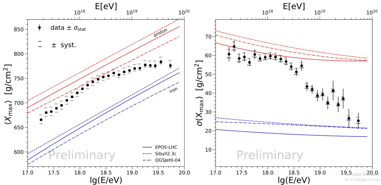
Figura 5.6.1: Evolución del valor medio de X_{max} (izquierda) y sus fluctuaciones (derecha) en función de la energía primaria, medido por el Observatorio Pierre Auger. Se observan las curvas teóricas de los modelos hadrónicos acotando el comportamiento entre protón (líneas rojas superiores) y hierro (líneas azules inferiores). Se ve también la dependencia lineal que hay entre el X_{max} y el logaritmo de la energía del primario. Extraído de [36].
