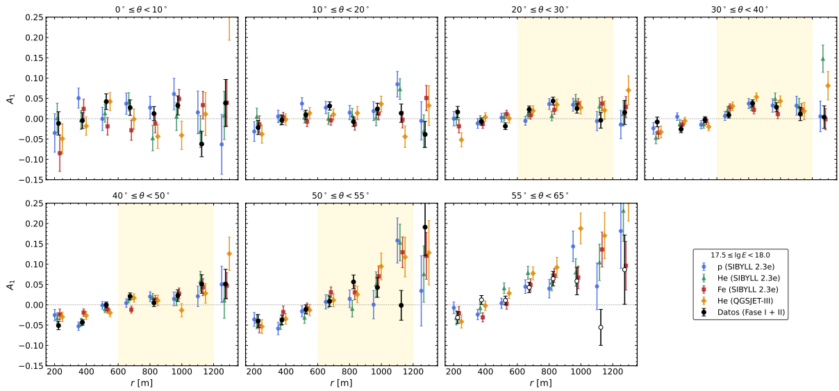
Figura 6.4.3: A_1 en función de la distancia al núcleo reconstruido, por banda de ángulo cenital reconstruido, para 17,5 \leq \lg(E/\text{eV}) < 18,0 . Negro: datos de campo (Fase I + II). Colores: simulaciones reconstruidas de protón, helio y hierro (SIBYLL 2.3e) y de helio (QGSJET-III), desplazadas levemente en r para facilitar la lectura. La franja sombreada marca la región 600 \leq r < 1200\text{ m} y 20^\circ \leq \theta < 55^\circ . En la banda 55^\circ \leq \theta < 65^\circ los datos se muestran con símbolos vacíos.
