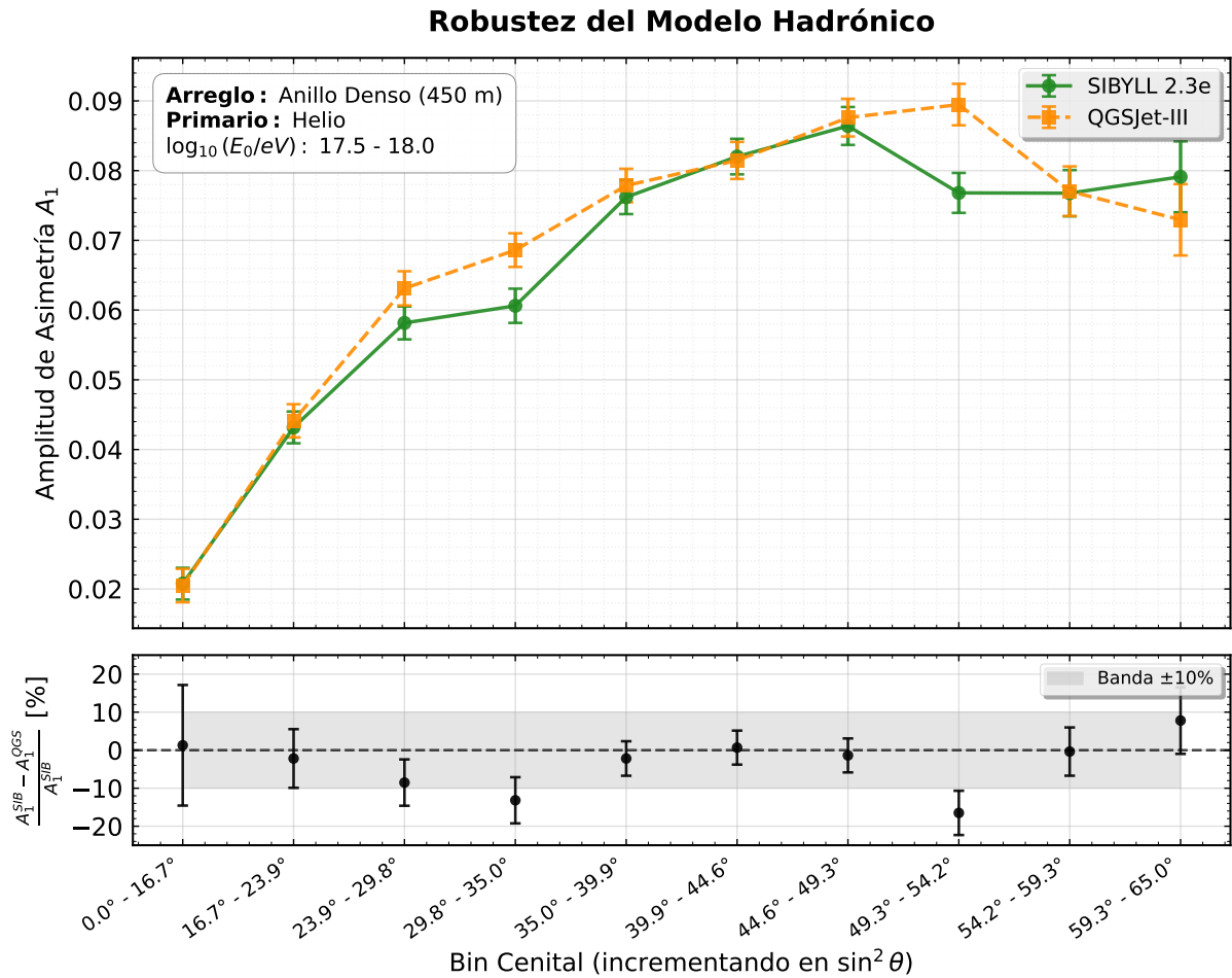
Figura 5.3.2: Comparación de la amplitud A_1 para lluvias de Helio simuladas con diferentes modelos hadrónicos. El panel inferior muestra que la diferencia relativa se mantiene mayoritariamente dentro de una banda de tolerancia aceptable, indicando una tendencia común independiente del modelo.
