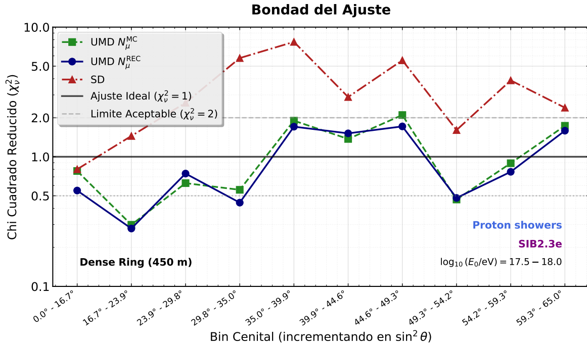
Figura 5.2.1: Bondad de ajuste \chi_\nu^2 para los bins cenitales. Se observa que los ajustes del UMD (REC y MC) se mantienen cercanos a la unidad, mientras que el SD presenta valores elevados debido a la alta precisión estadística de la muestra.
