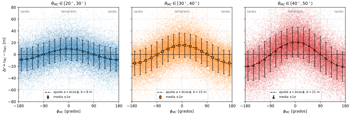
Figura 5.2.5: Error radial \Delta r = r_{MC} - r_{REC} de las estaciones del Infill en función de su azimut en el plano de la lluvia, para tres intervalos de ángulo cenital (protones, SIBYLL 2.3e, 17,5 \leq \log_{10}(E/\text{eV}) < 18,0 ). Cada punto es una estación; los marcadores son la media en cada intervalo de azimut, con barras de \pm 1\sigma (la dispersión de las estaciones; el error de la media es menor que el marcador), y la curva a trazos es el ajuste a + b \cos \phi . La modulación en coseno muestra que el núcleo reconstruido no sufre un esparsamiento aleatorio, sino un corrimiento sistemático de tamaño b hacia la región temprana.
