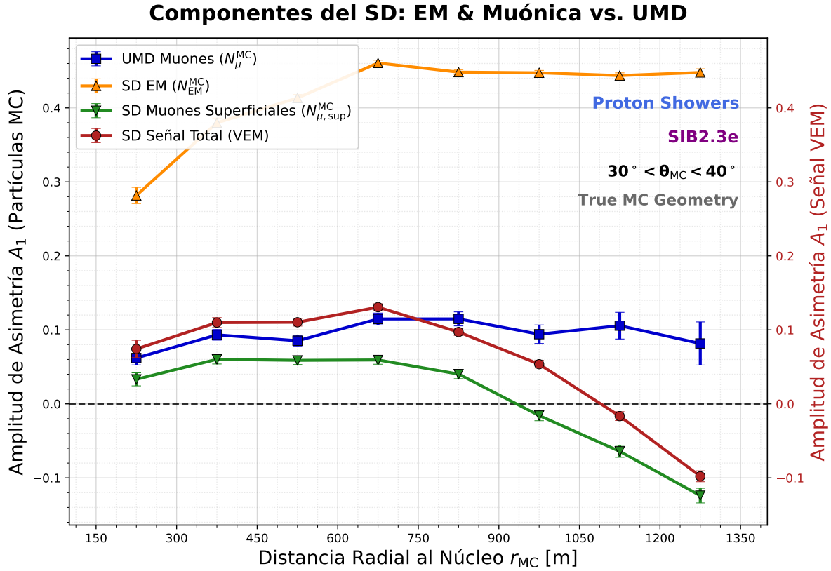
Figura 6.1.4: Desglose de la asimetría azimutal para las componentes inyectadas a nivel del suelo frente al número de muones inyectado en el detector subterráneo ( N_{\mu}^{MC} ), para 30^{\circ} \leq \theta < 40^{\circ} y geometría Monte Carlo. La asimetría electromagnética del SD (naranja) exhibe un comportamiento marcadamente positivo acoplado a la evolución longitudinal. En contraste, los muones del SD (verde) presentan una asimetría negativa a grandes distancias cuando se calcula sobre las estaciones que forman parte del evento reconstruido (Sección 6.1.3). Las barras de error representan el error estándar de la media.
