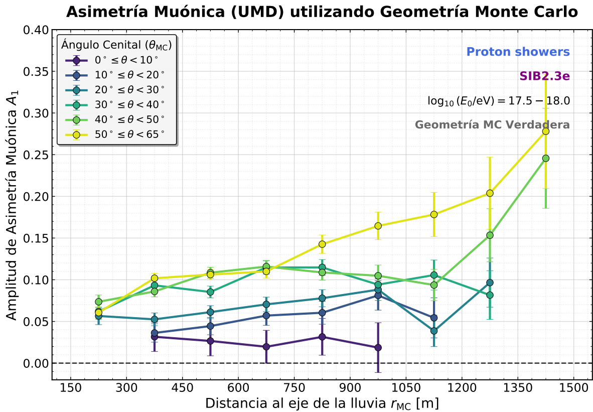
Figura 6.1.1: Evolución de la amplitud de asimetría A_1 en función de la distancia al núcleo para distintos rangos de inclinación cenital. El análisis utiliza la geometría verdadera (Monte Carlo) y un bineado radial dinámico ajustado a la viabilidad estadística de cada régimen.
