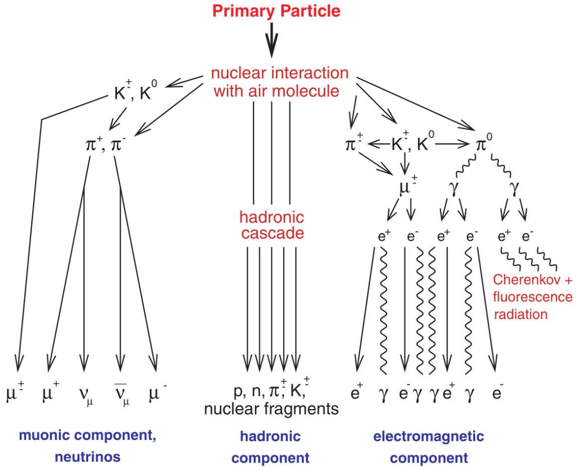
Figura 1.2.1: Imagen esquemática del esqueleto hadrónico que caracteriza a las lluvias atmosféricas extensas. Obtenido de [11].
