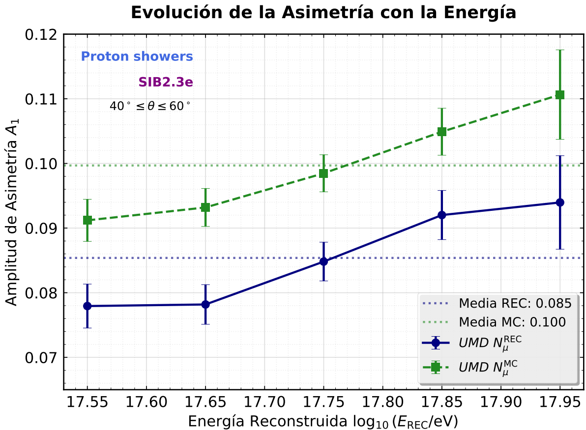
Figura 5.4.1: Evolución de la amplitud de asimetría A_1 en función de la energía reconstruida para cascadas de protón simuladas con SIBYLL 2.3e. Se observa un leve incremento lineal en la asimetría a mayores energías, presente tanto a nivel Monte Carlo como en la reconstrucción.
