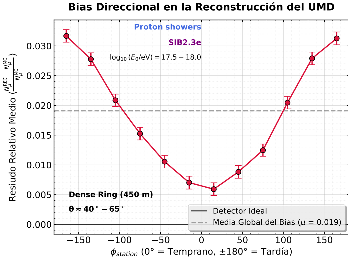
Figura 5.2.3: Distribución de la media del residuo relativo de reconstrucción en función del ángulo azimutal de la estación en el plano de la lluvia. Se evidencia un desempeño degradado en las regiones tardías ( \pm 180^\circ ), donde el sesgo de sobreconteo es máximamente superior al de la región temprana ( 0^\circ ).
